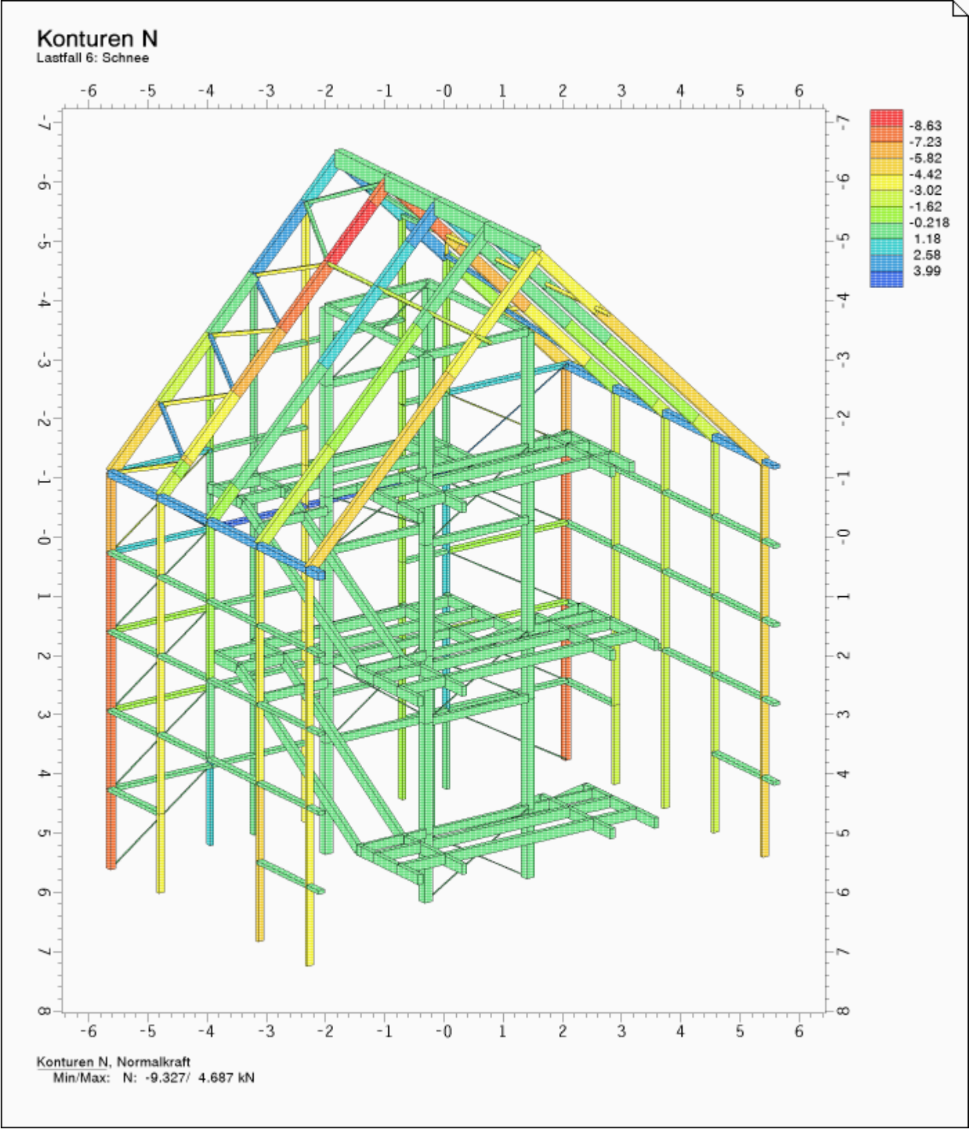
Druckfragment Lastfallergebnisse
