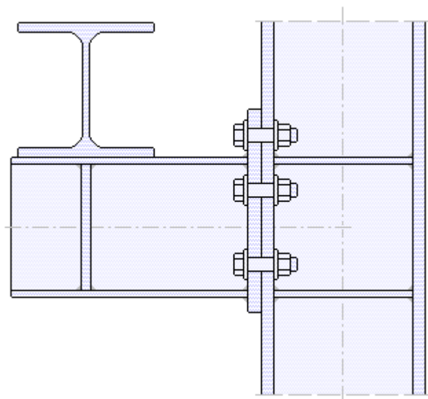
Anschluss links - geschraubt - Steifen
