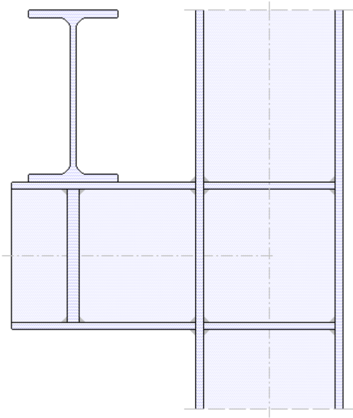
Anschluss links - geschweißt - Lastträger - Steifen
