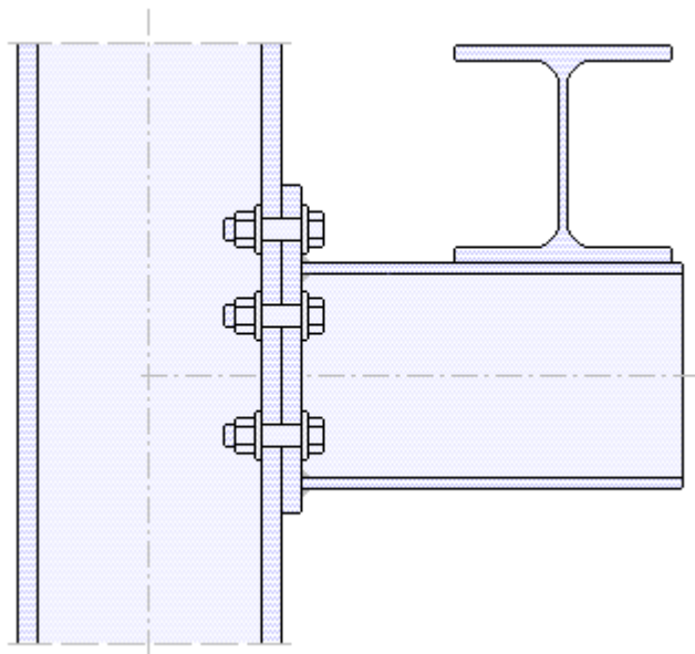
Anschluss links - geschraubt - Steifen
