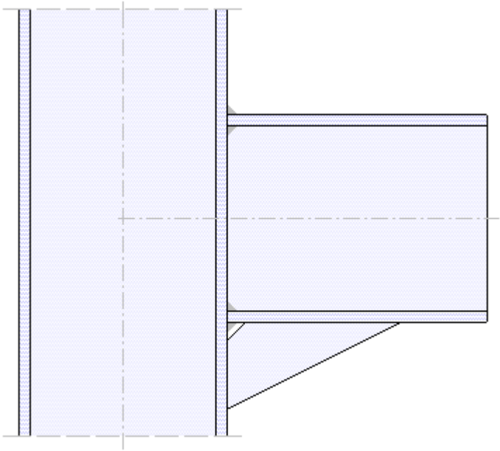
Anschluss links - geschweißt - Steifen - Voute
