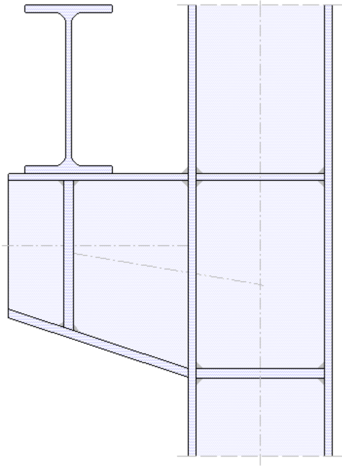
Anschluss links - geschweißt - Steifen - Voute
